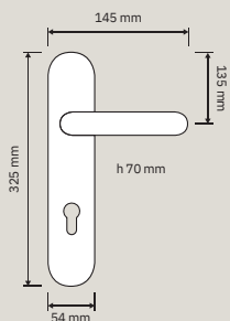
1307 MN 232 Maniglione / Pull handle
